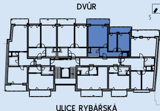
PŮDORYS 3.NP
