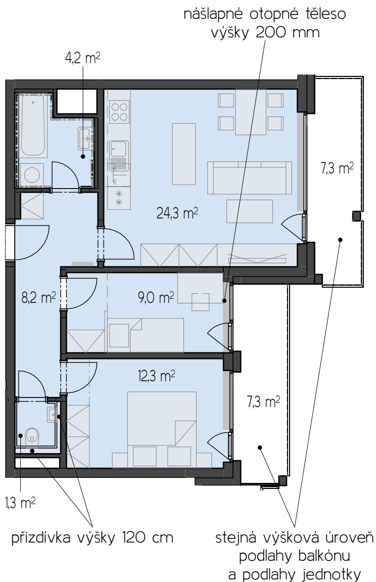
PŮDORYS 6.NP
