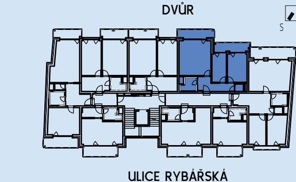
PŮDORYS 7.NP
